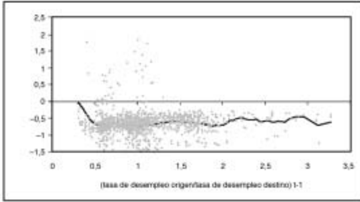
Gráfico 2. Variable no paramétrica ECU-1 -m\left(\frac{u_i}{u_j}\right)_{t-1}
