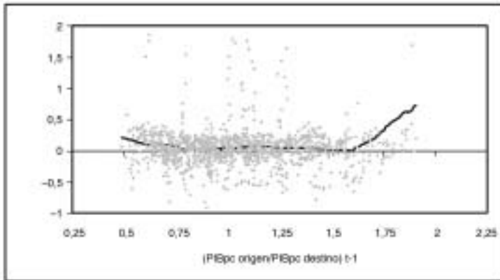
Gráfico 3. Variable no paramétrica ECU-2 -m\left(\frac{Y_i}{Y_j}\right)_{t-1}
